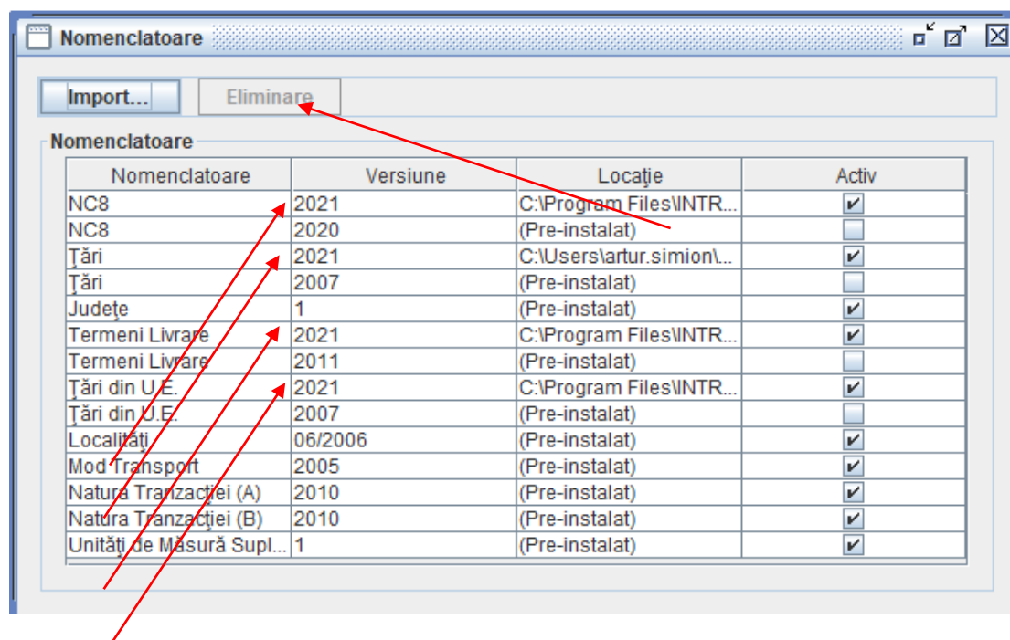
Figura 1 . Administrare nomenclatoare - eliminarea nomenclatoarelor NC 2021, țări din UE, țări de origine și termeni de livrare.
