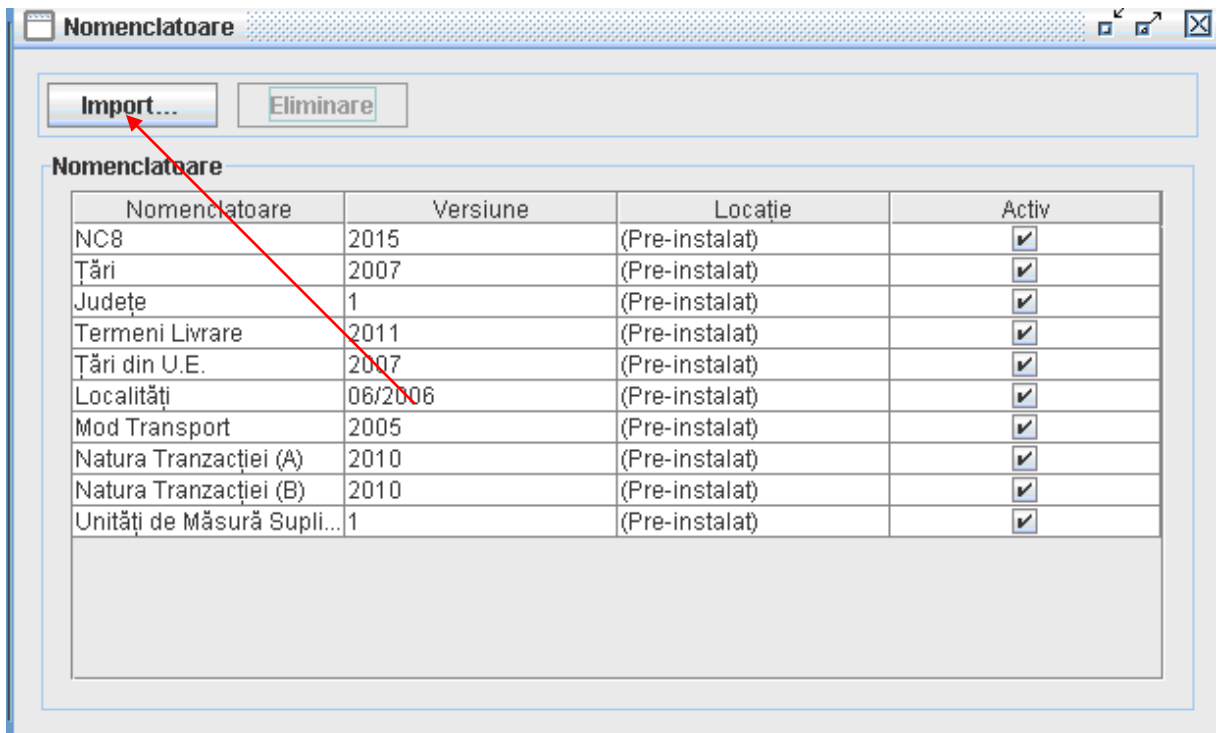
Figura 20. Administrare nomenclatoare
